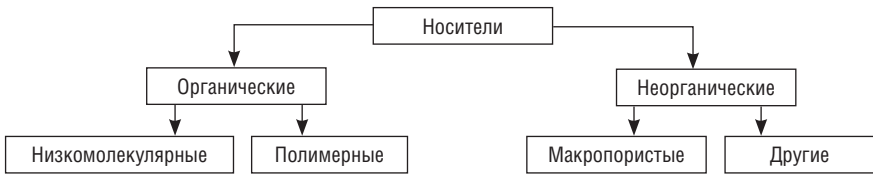
Рис. 6.1. Классификация носителей для иммобилизации ферментов
