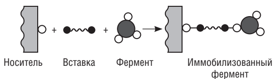
Рис. 6.3. Схема иммобилизации фермента химическим методом
