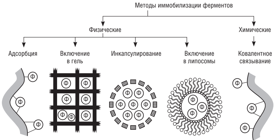
Рис. 6.2. Методы иммобилизации ферментов: \Phi — молекула фермента
