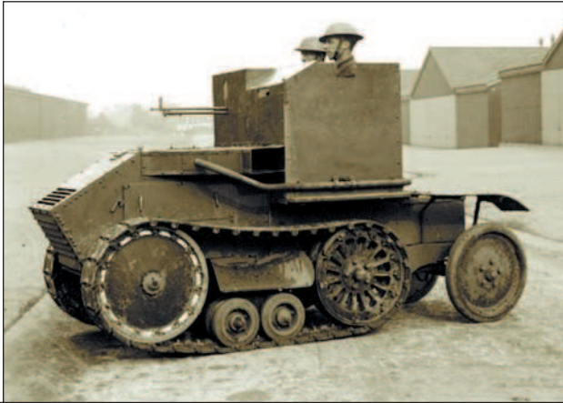
Танкетка «Моррис-Мартель» двухместного типа, мод. 1927 г.
