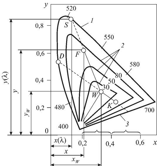
Рис. 1.1. Цветовой график МКО для определения характеристик цвета: 1 — линия спектральных цветов; 2 — линии постоянной чистоты; 3 — линия «чистых» пурпурных цветов
