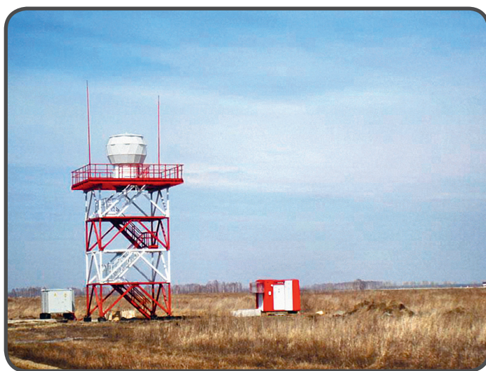
Фото 1.6. Радиолокатор обзора летного поля «Атлантика ЭЗ»
