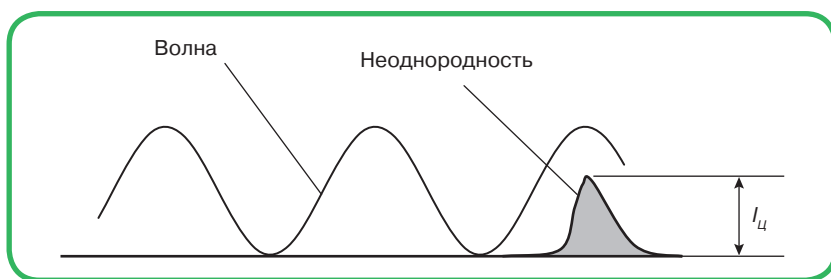
Рис. 2.14. Графическая иллюстрация ситуации, при которой радиоволна не отражается от цели
