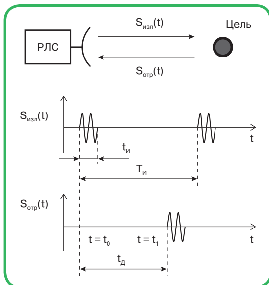
Рис. 2.2. Измерение дальности до цели с помощью радиоволн
