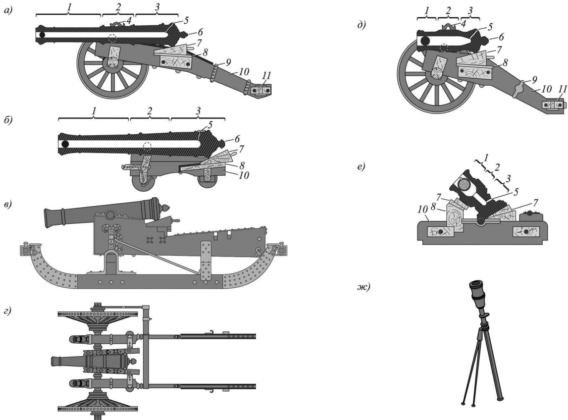
Артиллерийские орудия: а) полевая пушка на колёсном лафете; б) корабельная пушка; в) полковая пушка на лафете-санях; г) полковая пушка с двумя мортирами на лафете конструкции В.Д. Корчмина; д) гаубица на колёсном лафете; е) мортира; ж) ручная мортира на треножном станке. Цифрами обозначены: 1 – дульная часть ствола; 2 – вертлюжная часть ствола; 3 – казённая часть ствола; 4 – дельфин; 5 – запальное отверстие; 6 – винград; 7 – подъёмный клин; 8 – подклиновья подушка; 9 – оковка лафета; 10 – станина лафета; 11 – хоботовая подушка
