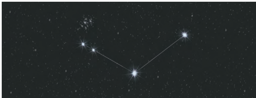
Созвездие Гончие Псы.
