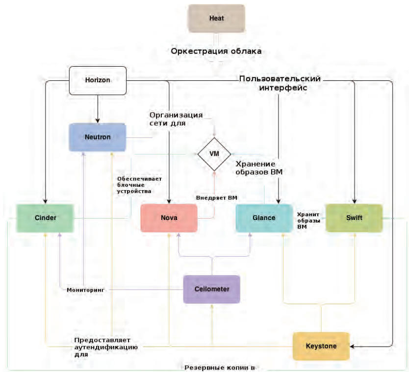
Рис. 1.2 ❖ Архитектура OpenStack
