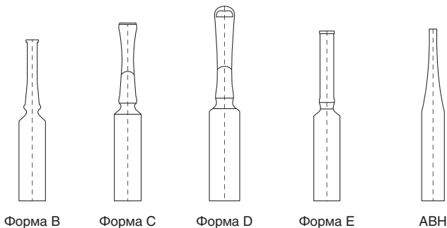
Рис. 1.3. Разновидности геометрии ампул: формы В, С, D, E — для шприцевого наполнения; АВН — для вакуумного наполнения
