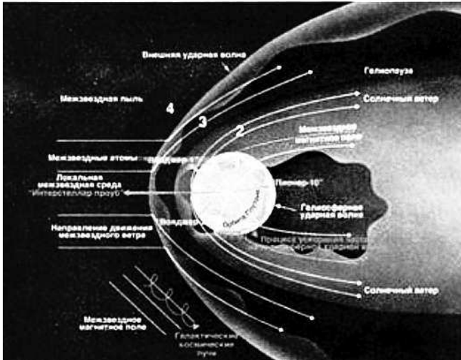
Рис. 6. Водородный пузырь Солнечной системы — гелиосфера
