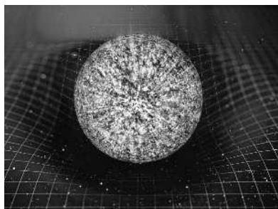
Рис. 1. Солнце в сетке пространства
