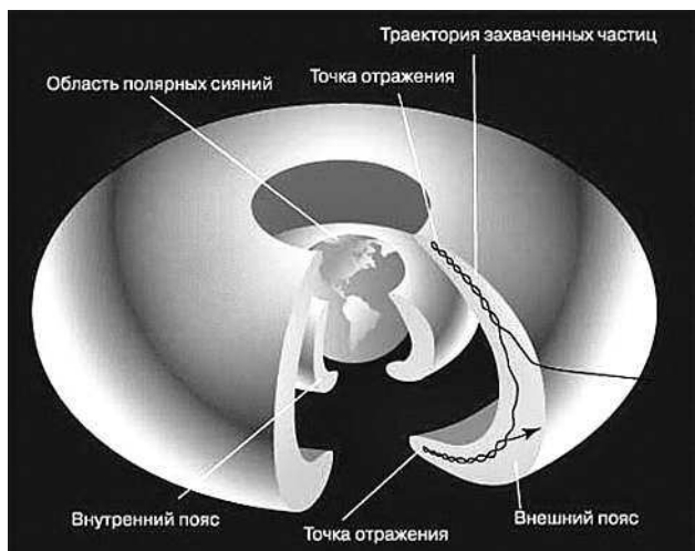
Рис. 5. Пояса Ван Аллена
