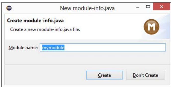
Рис. 1.25. Создание модуля
