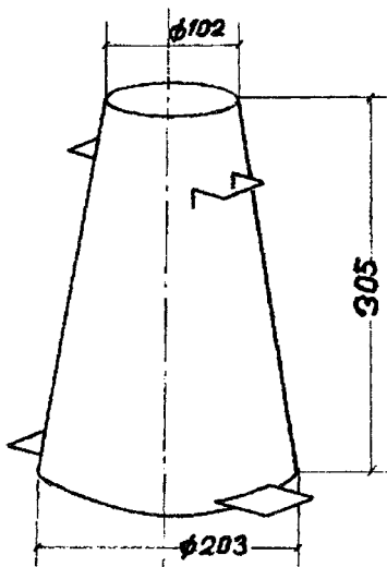
Рис. 2. Конус для определения пластичности бетона
