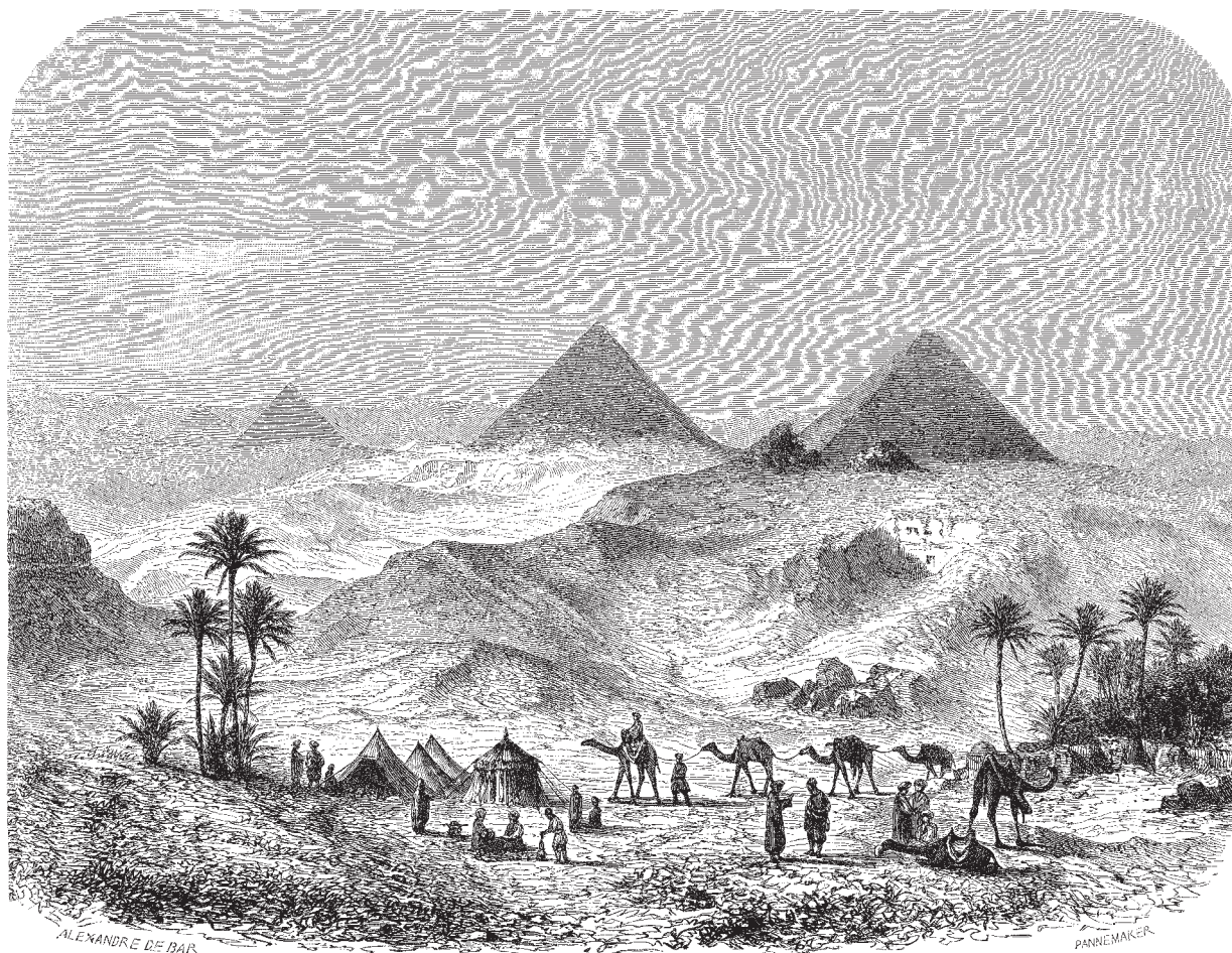
Рис. 5. Пирамиды
