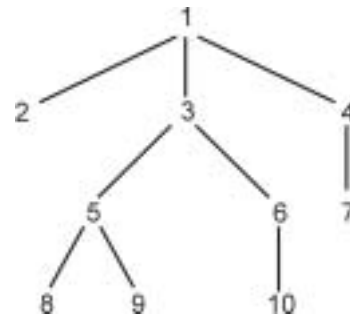
Рис. 3.3. Дерево
