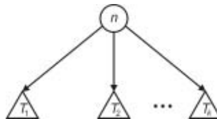
Рис. 3.4. Дерево T
