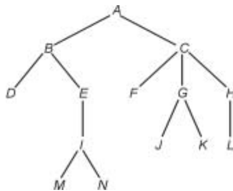
Рис. 3.18. Дерево
