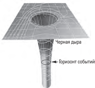
Рис. 52. Горизонт событий
