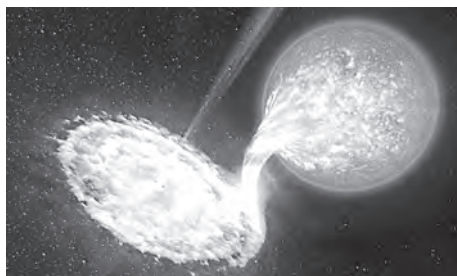
Рис. 48. Поглощение звезды черной дырой (см. рис. 5 на цветной вклейке)
