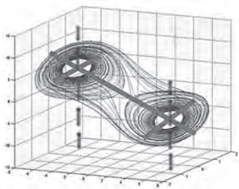
Рис. 50. Аттрактор и оптические коридоры
