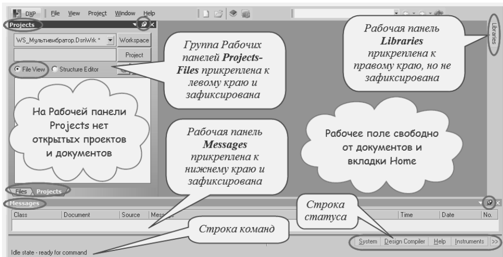
Рис. 1.19. Стартовое состояние окна системы
