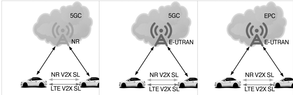
Рис. 1.4. Сценарии линии боковой связи SL с использованием радиointерфейса NR
