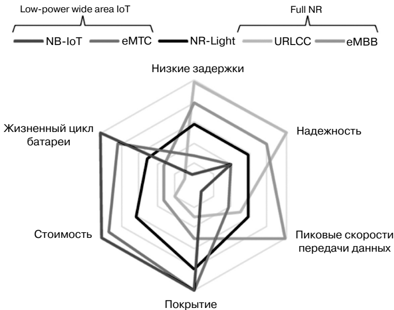
Рис. 1.3. Сравнение характеристик NR Light
