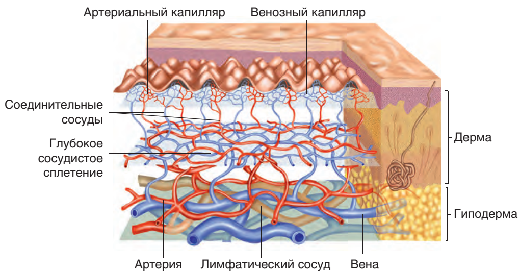
Рис. 1.3. Схема строения и расположения в коже кровеносных и лимфатических сосудов
