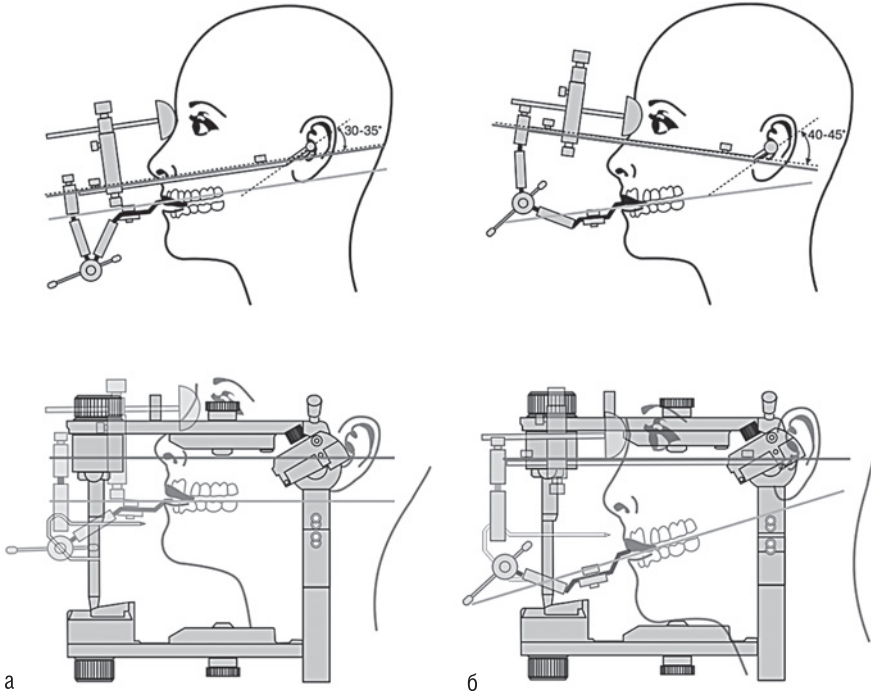
Рис. 1.2.7. Установка лицевой дуги по камперовской плоскости (а) и по франкфуртской плоскости (б)
