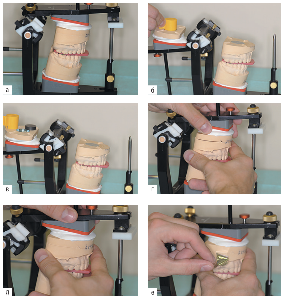
Рис. 1.2.12. Контроль точности заливки моделей: а — гипсовые модели установлены в артикулятор с межокклюзионным восковым регистратом; б — извлечение магнита из отдельного цоколя модели верхней челюсти; в — подготовленные к проверке модели с извлеченным магнитом; г — проверка точности заливки — цокольные части точно не совпадают (ошибка монтажа модели нижней челюсти); д — проверка точности заливки — совпадение цокольных частей модели (корректный монтаж модели нижней челюсти); е — проверка плотности смыкания цокольных частей артикуляционной фольгой (без красителя) толщиной 12 мкм
