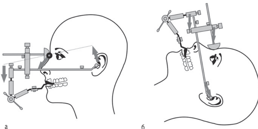
Рис. 1.2.9. Наложённая на голову пациента анатомическая лицевая дуга в вертикальном (а) и горизонтальном (б) положении
